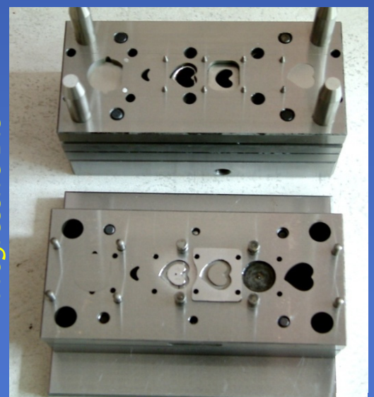
Progressive Die
